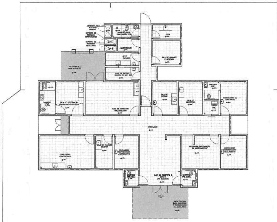
Planta Baixa Acabamento Piso Esc. 0/08
